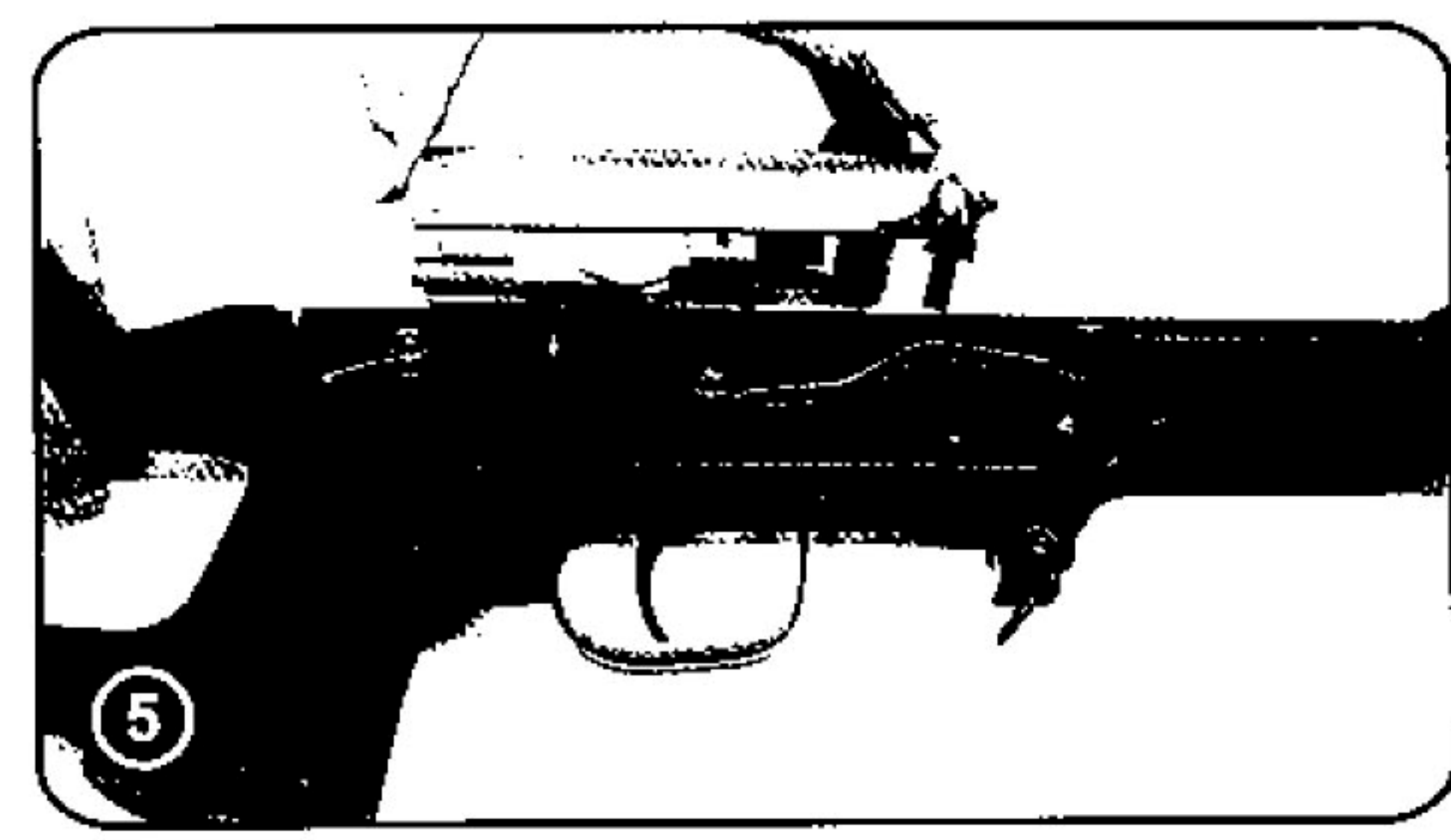
取出槍機
