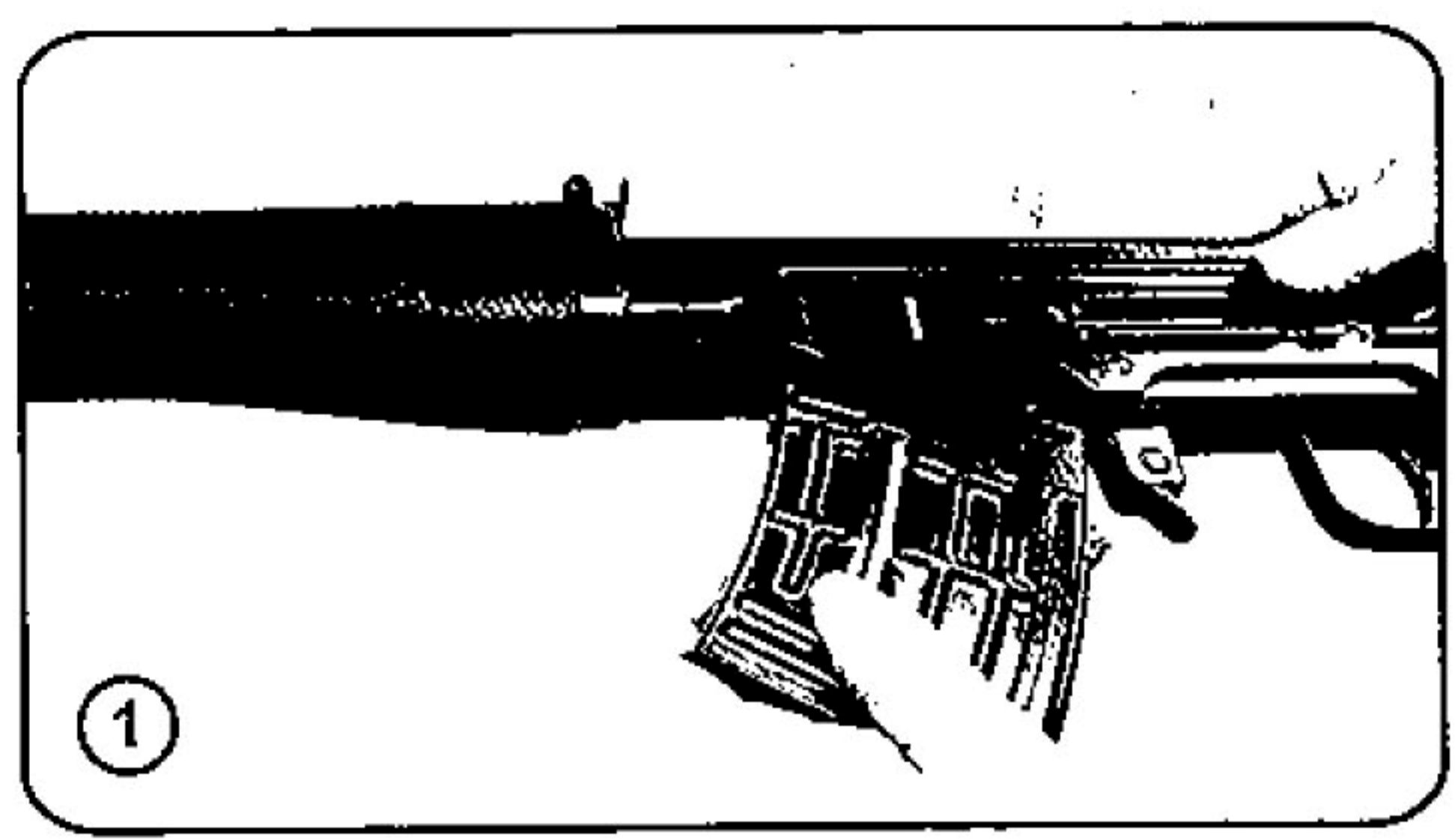
取下彈匣，拉拉柄確認槍膛內有無子彈，關保險
