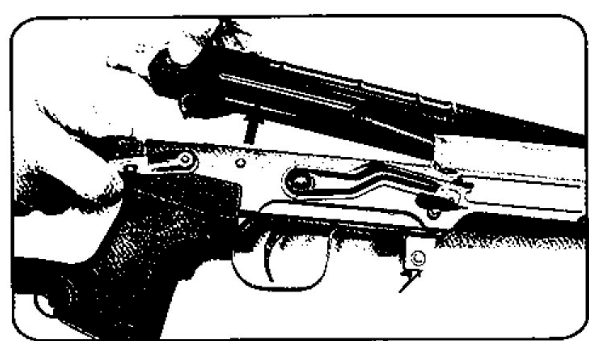
掀開上蓋，並取出復進彈簧桿
