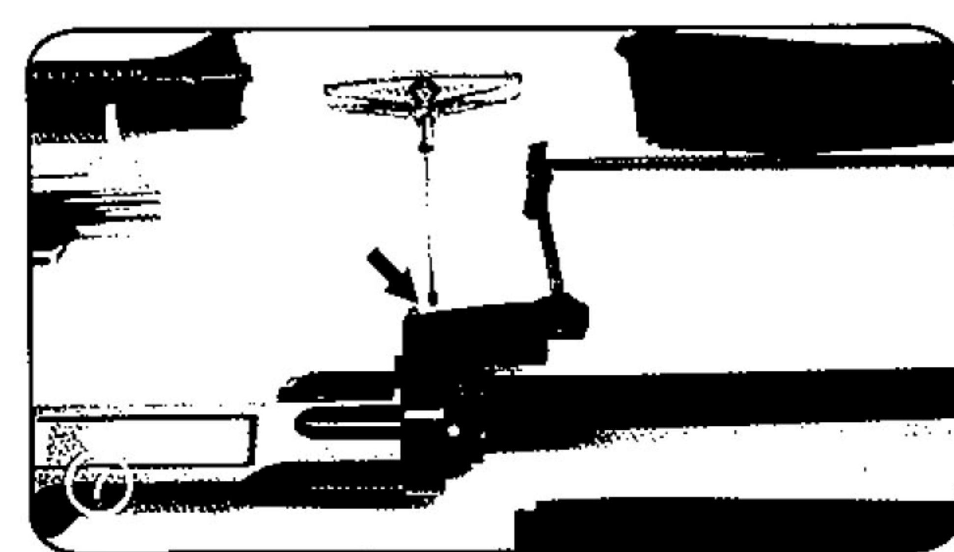
如需拆卸槍管，需取出瓦斯鋼管套組及取出微調螺絲、左右螺絲、插銷
