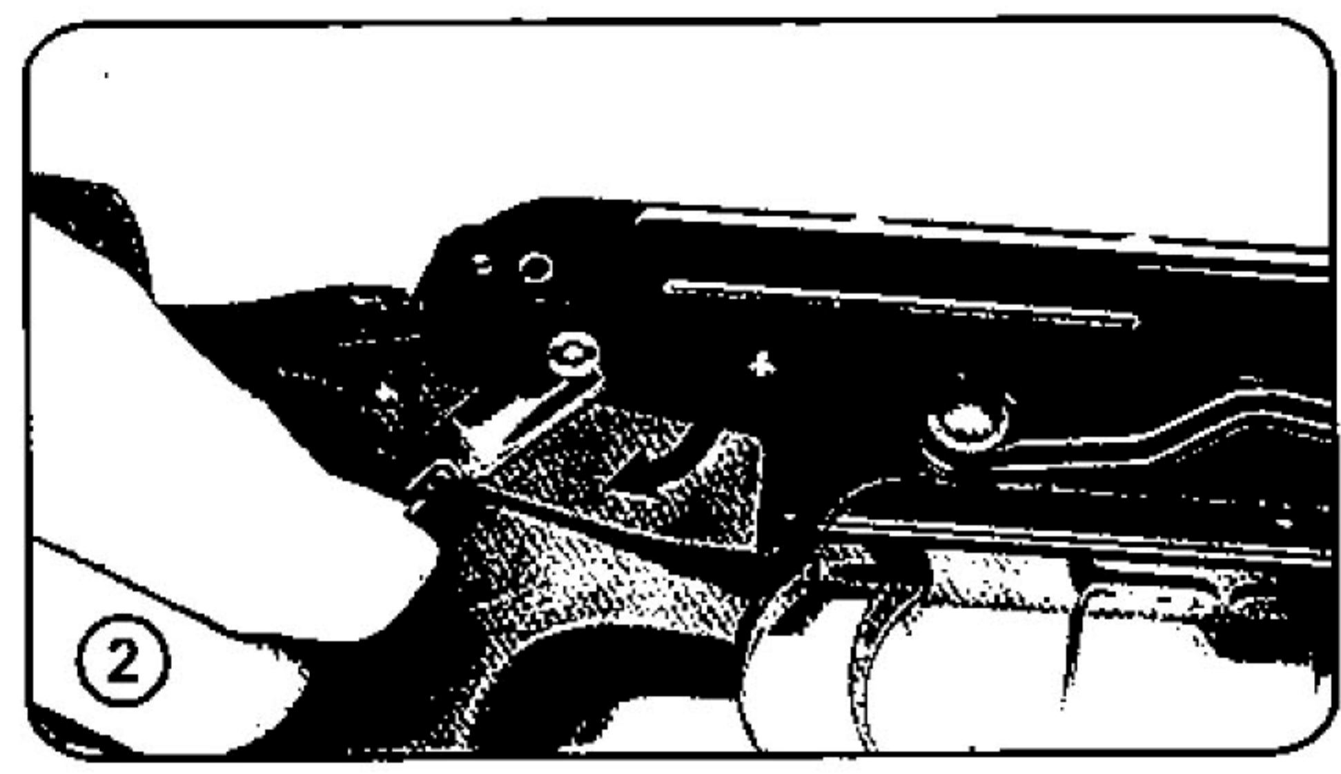
將上蓋固定器往後至固定鈕位置，上蓋即可掀開
