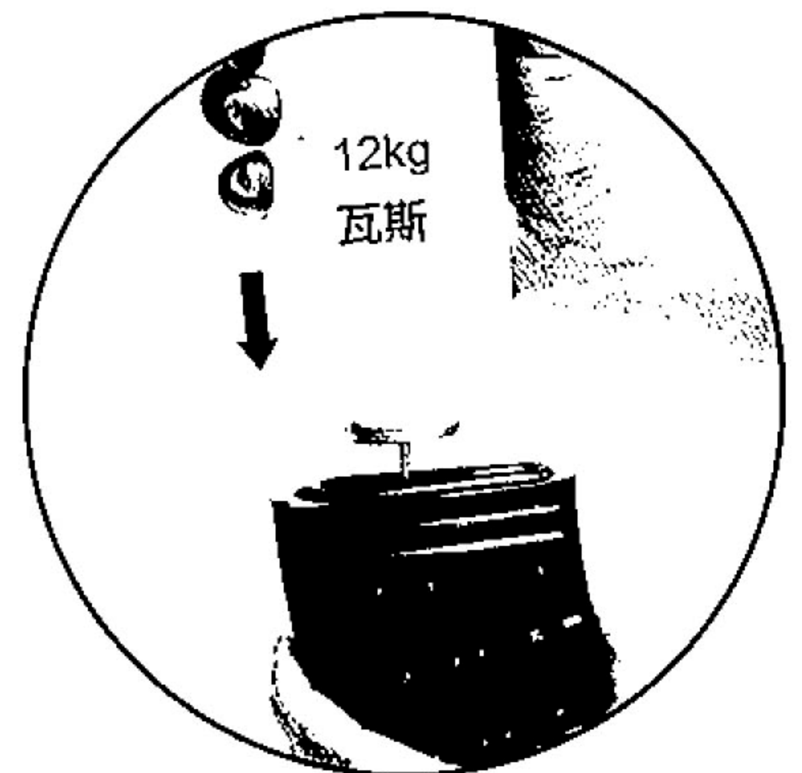
將瓦斯由底版注入孔灌入 Fill gas from bottom of magazine. ※限使用12kg 瓦斯 (R22/Green Gas)
